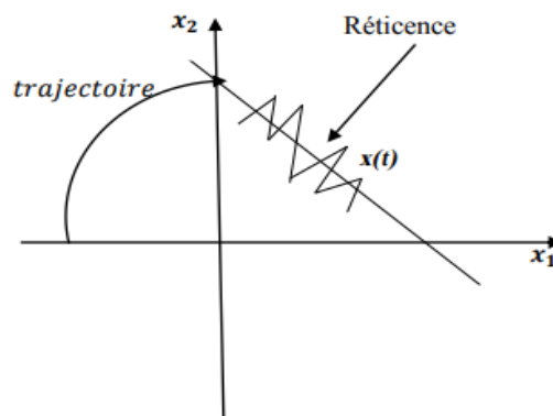
Figure (III.5) : Phénomène de chattering (réticence) [51].
