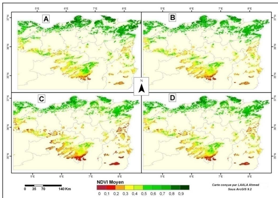
Fig.10 : NDVI saisonnier moyenne calculé pour la période (2002-2011) au cours de l'hiver (A), le printemps (B), l'été (C) et l'automne (D)
