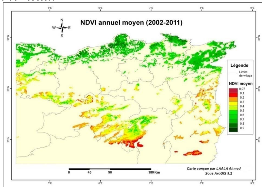
Fig.6 : NDVI annuel moyen calculé pour la période (2002-2011)
