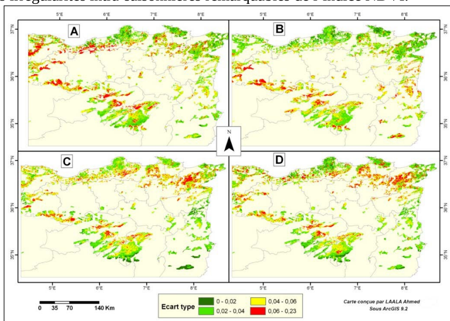
Fig.11 : Ecart type intra-saisonnier d'NDVI calculé pour la période (2002-2011) au cours de l'hiver (A), le printemps (B), l'été (C) et l'automne (D)
