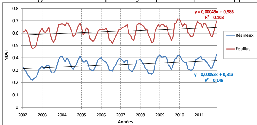
Fig.4 : Cycle annuel de la végétation forestière de l'Est algérien entre 2002 et 2011
