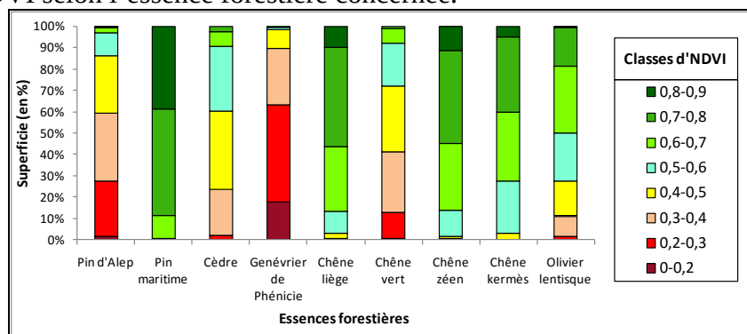
Fig.7 : Superficies (en %) de différentes classes d'NDVI pour chaque écosystème forestier
