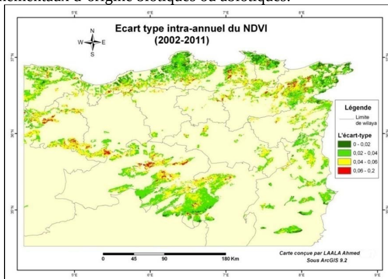
Fig.9 : Ecart type intra-annuel d'NDVI calculé pour la période (2002-2011)
