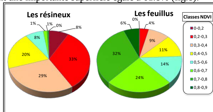
Fig.8 : Superficies (en %) de différentes classe d'NDVI pour la totalité des résineux et des feuillus de l'Est algérien
