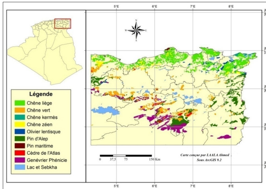
Fig.1. Principaux écosystèmes forestiers de l'Est algérien
