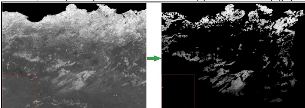
Fig.3 : Image satellitaire MODIS (acquise le 01/02/2002) avant et après l'application du masque
