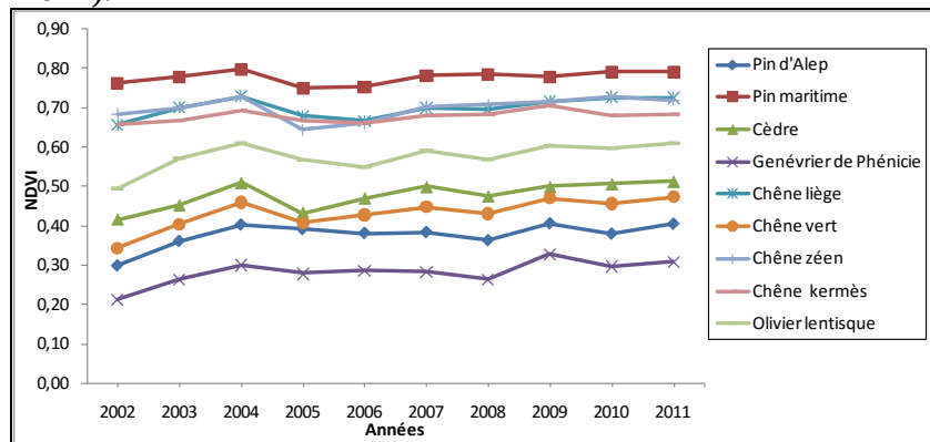
Fig.5 : Variation interannuelle de l'indice NDVI de différents écosystèmes forestiers étudiés
