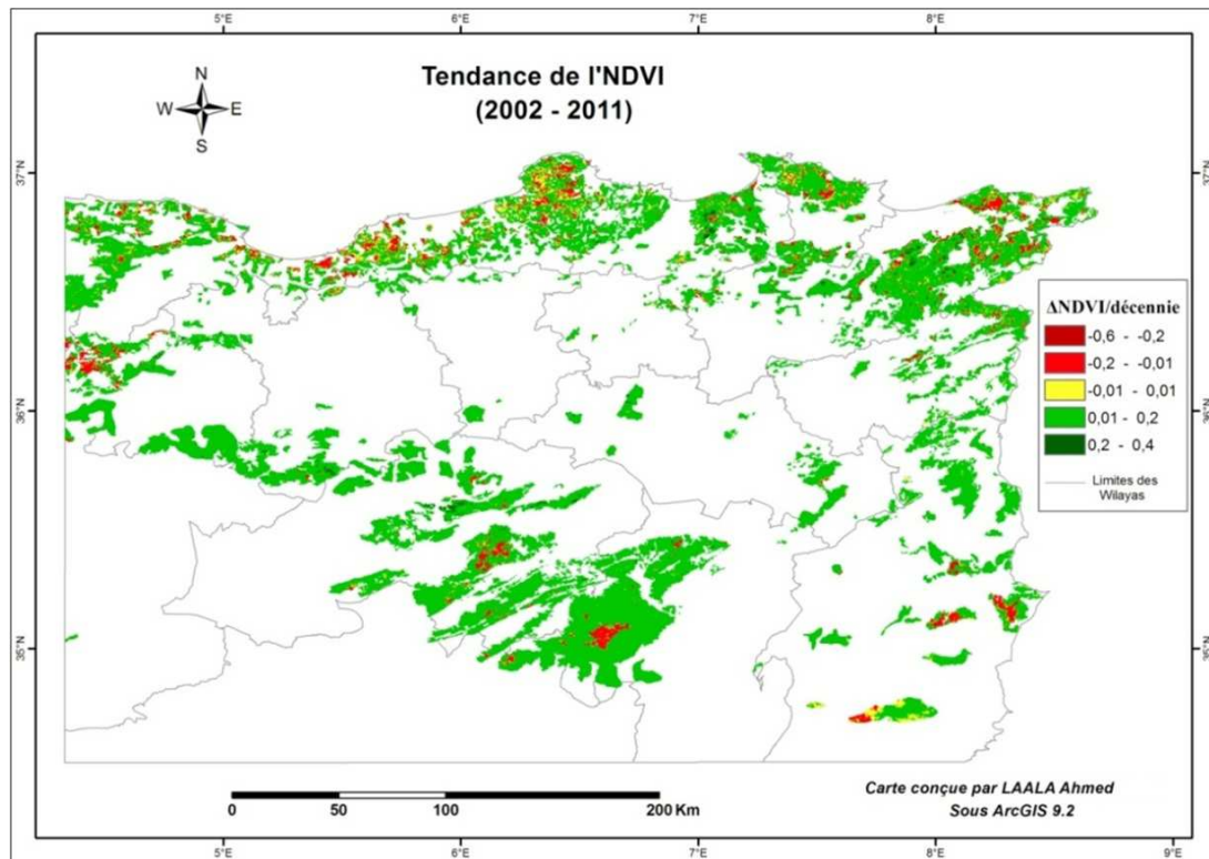
Fig.2. Tendance de l'indice NDVI sur la période 2002-2011
